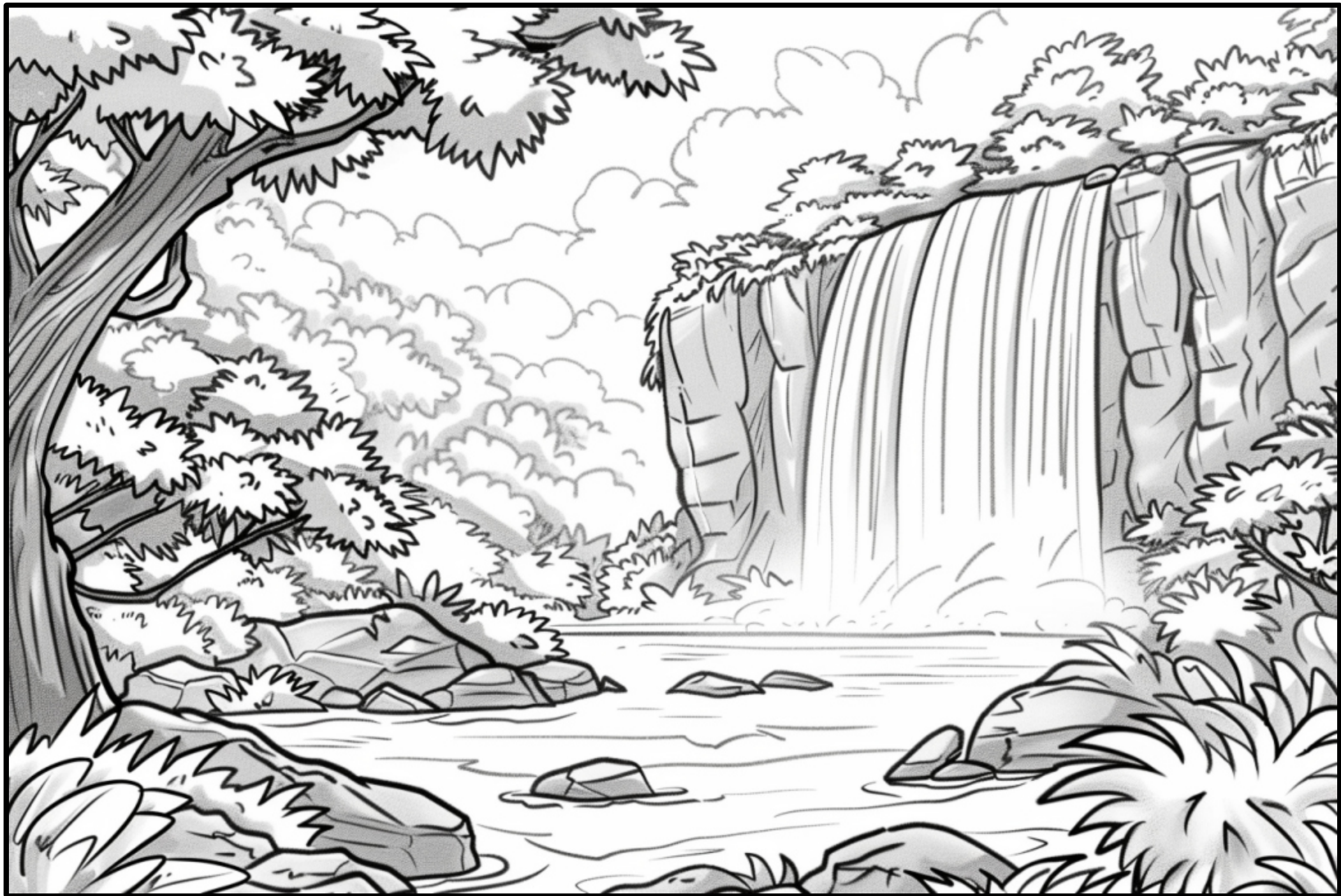
滝と溪谷
